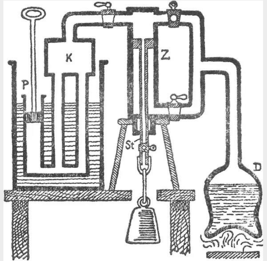
64) Watt's eerste model van een stoommachine met afzonderlijke condensator.
